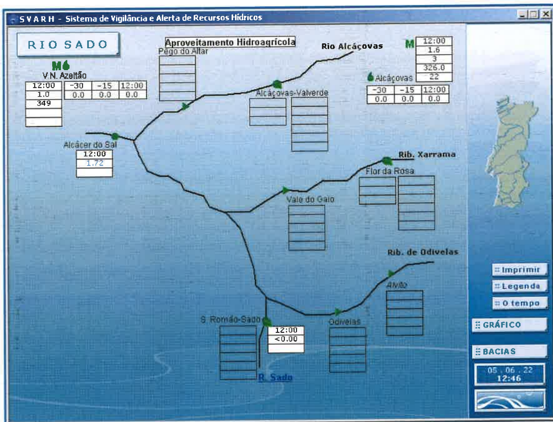
Figura 32 - Atual configuração do SVARH na RH, bacia do rio Sado
