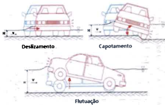
Figura 52 - Instabilidade causada em veículos em situação de inundação (Fonte: adaptado de Shand et Al., 2011)
