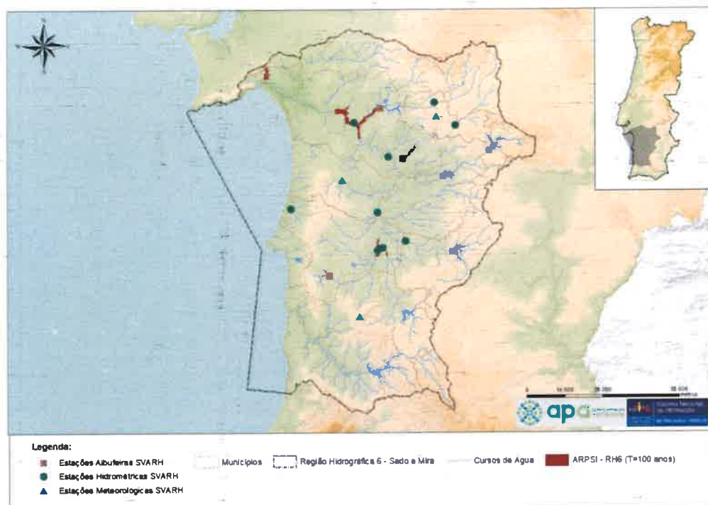
Figura 33 - Estações do SVARH na RH6
