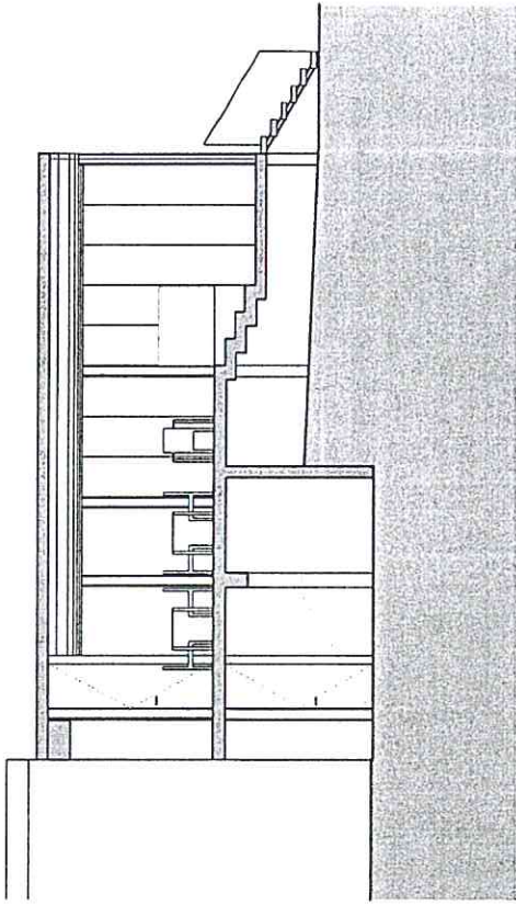
CORTE AA'
