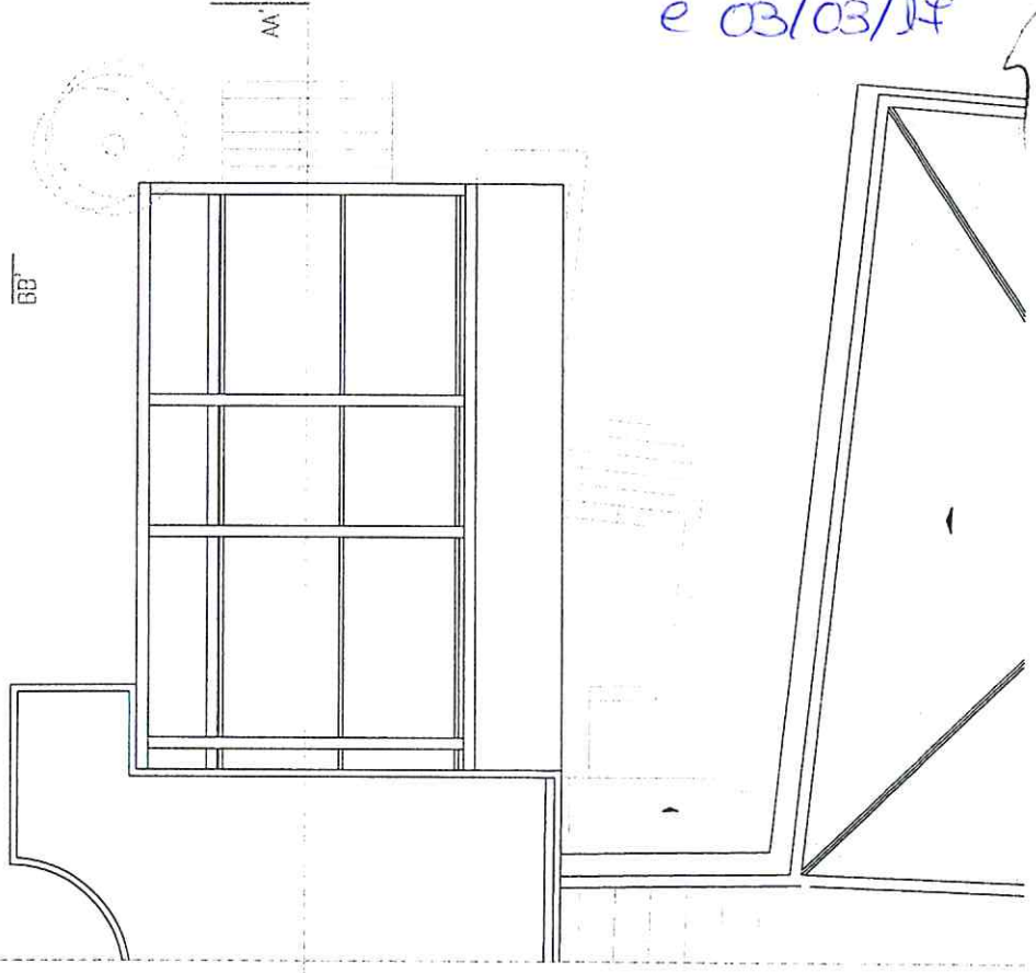
PLANTA DE ESTRUTURA DA COBERTURA
