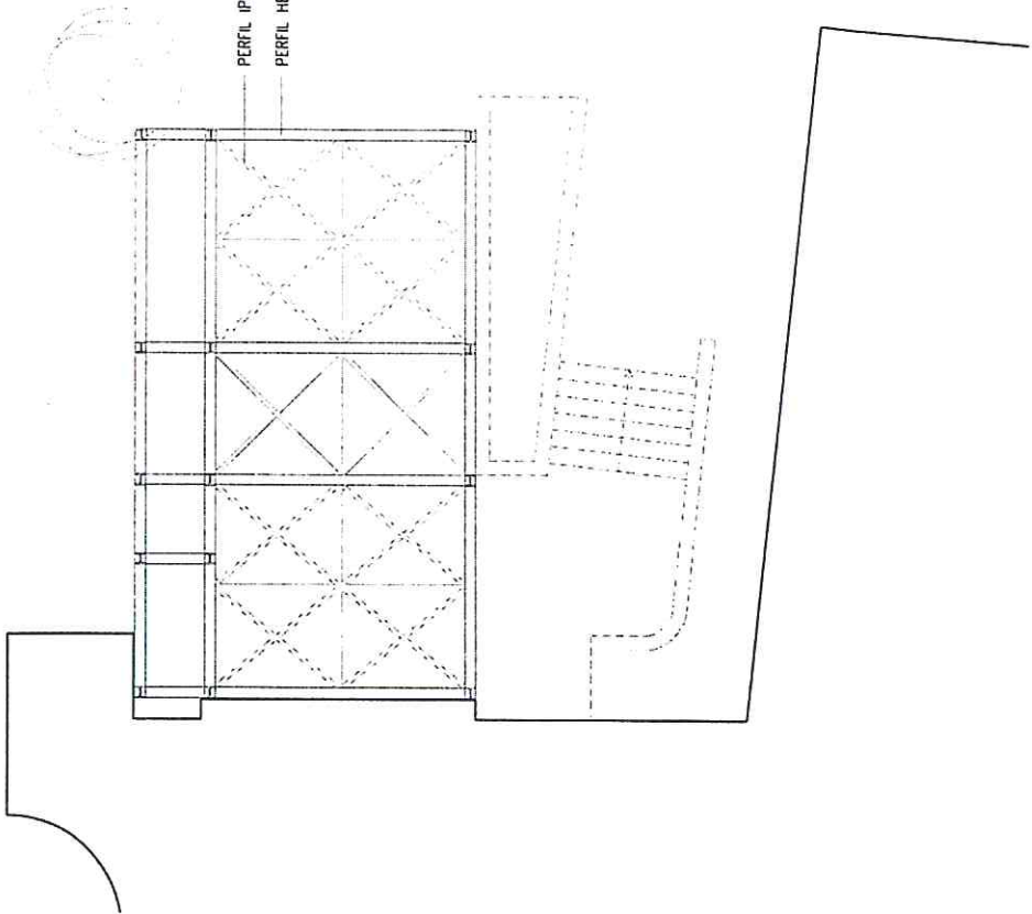
PLANTA DE ESTRUTURA DO PAVIMENTO
