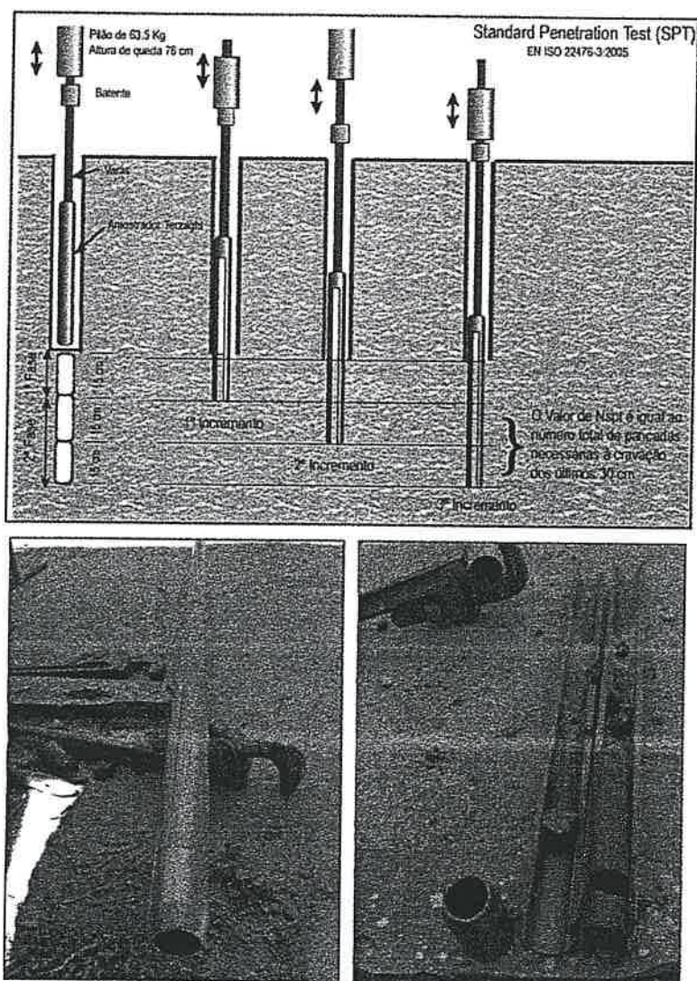
Figura 1 - Esquema de realização do ensaio SPT e respectivo equipamento
