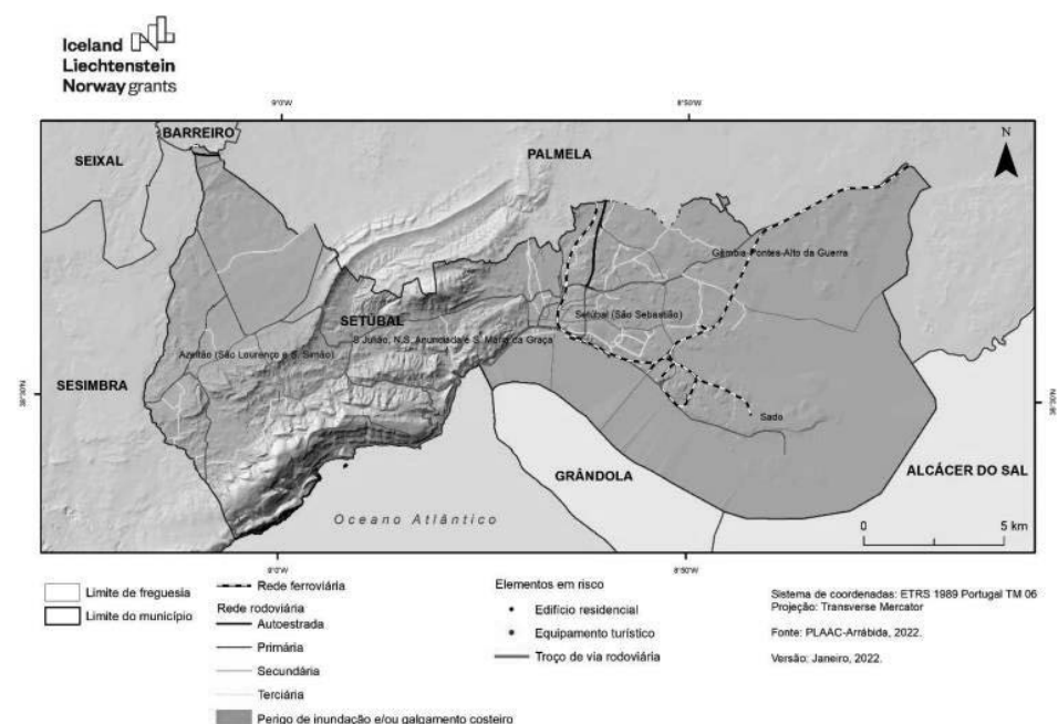
Figura 55. Elementos expostos em  reas suscetveis a inunda o e/ou galgamento costeiro no munic pio de Set bal.
