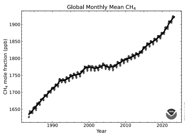
Figura 6. Média global da concentração de metano médio mensal na atmosfera determinado a partir de locais de superfície marinha desde 1983 a 2023.
